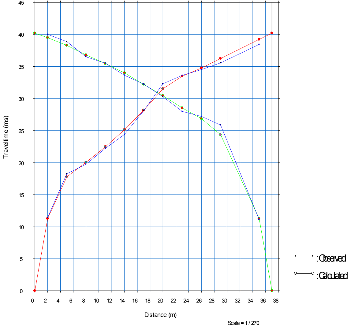
P Dalgası Yol-Zaman Grafiği
