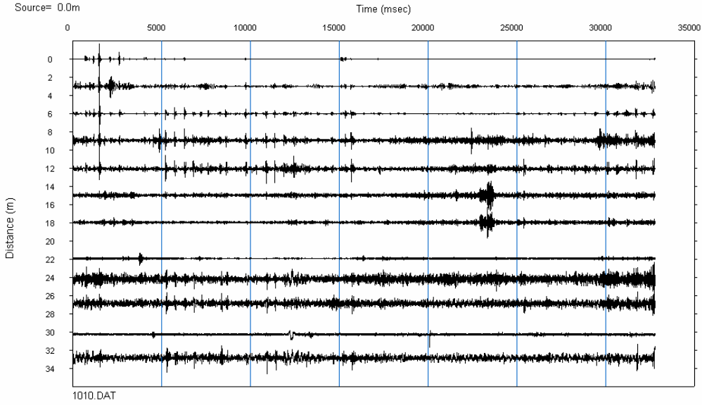
Mikrotremor Hattı Arazi Kaydı
