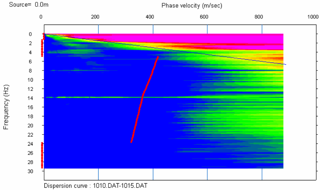
Dispersiyon Eğrisi
